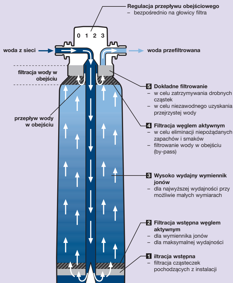
Schemat wkładu filtracyjnego BWT bestprotect z 5-stopniową filtracją
