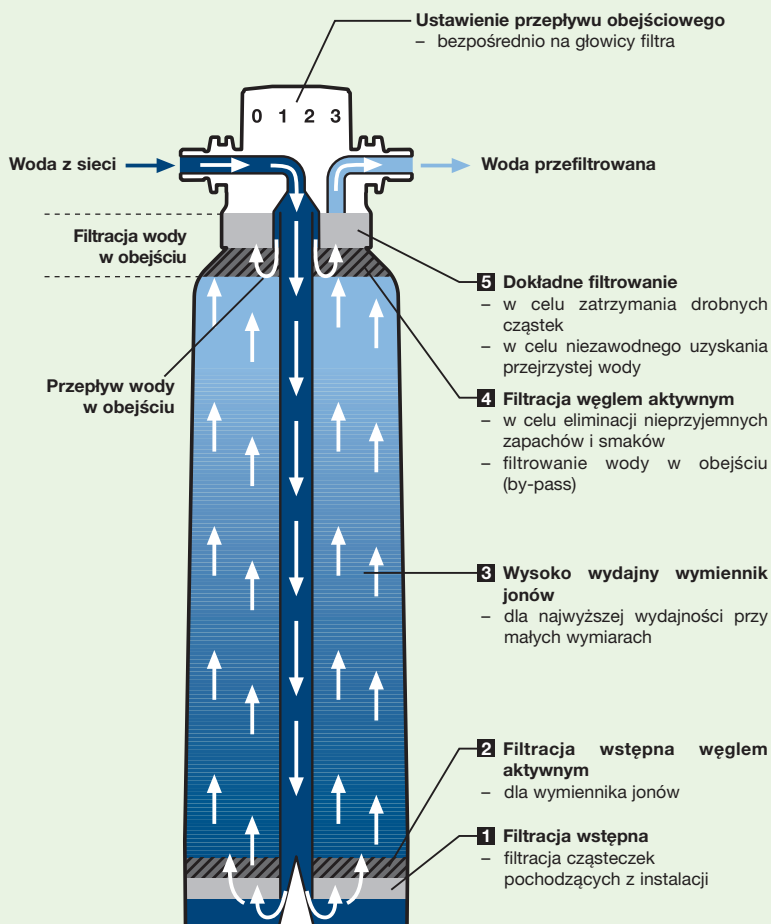
Budowa wkładu filtracyjnego BWT bestclear z 5-stopniową filtracją
